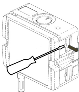
Figura 18 – Retirando a tampa do dispositivo (1)
