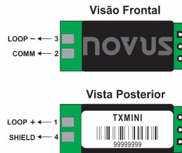
Figura 3 – Saída 4-20 mA
