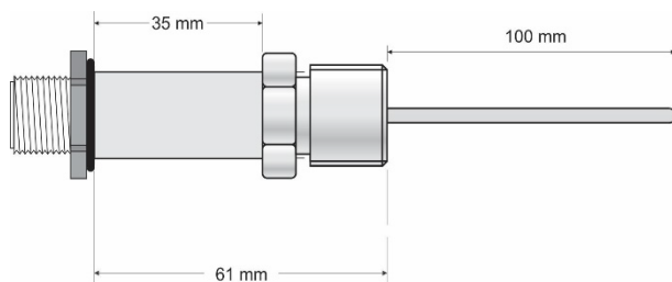
Figura 2 – Dimensões do transmissor TxMini-M12-MP
